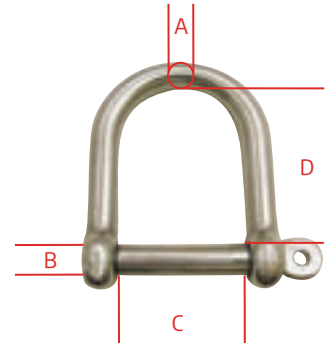
SSDS312
