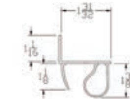
CP-07OF
