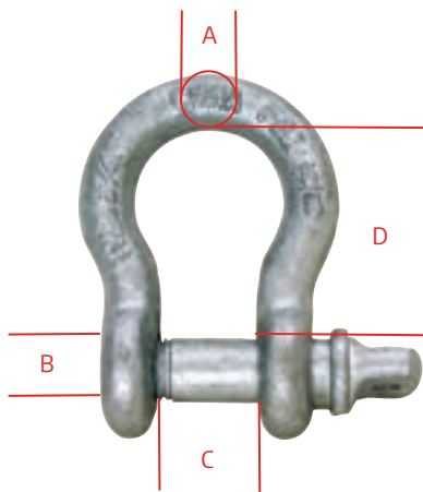
DRSPA625
