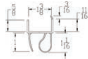
CP-05
