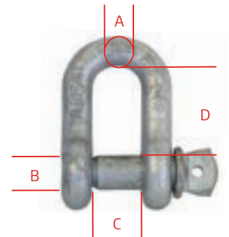
DRSPC375
